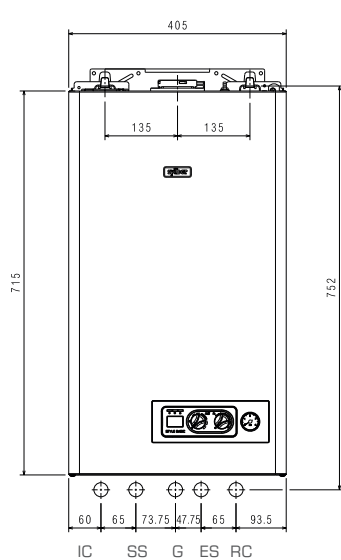
DISPOSICIÓN CONEXIONES
